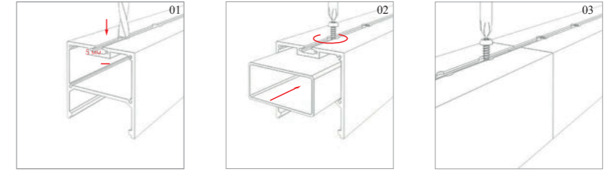
CON PROFILO DI ESTENSIONE
